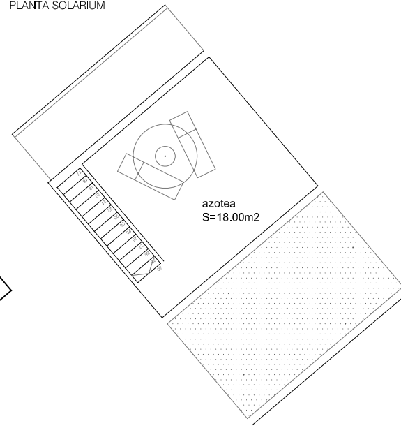
PLANTA SOLARIUM
