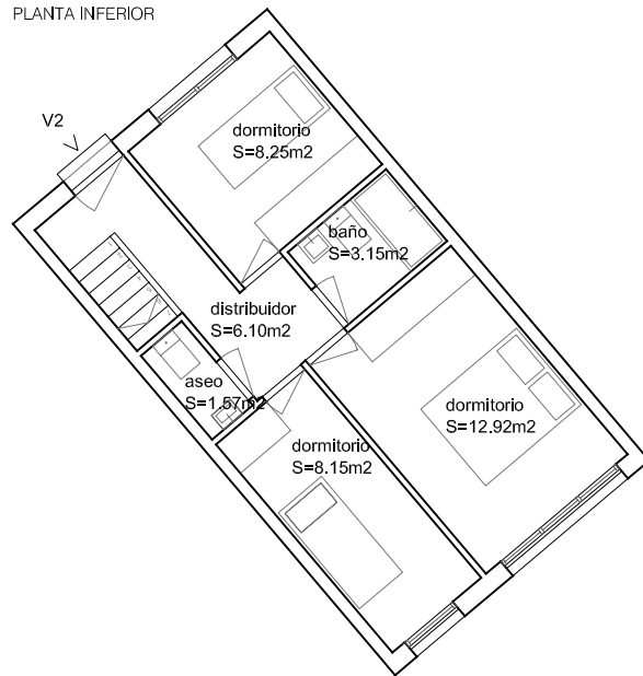
PLANTA INFERIOR
