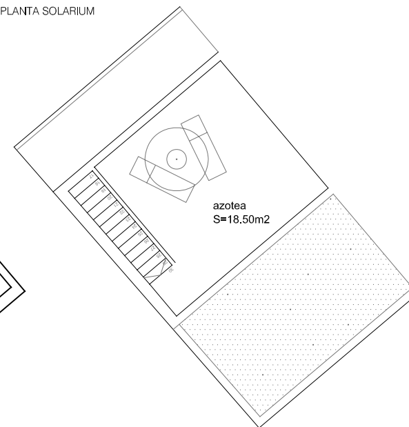
PLANTA SOLARIUM
