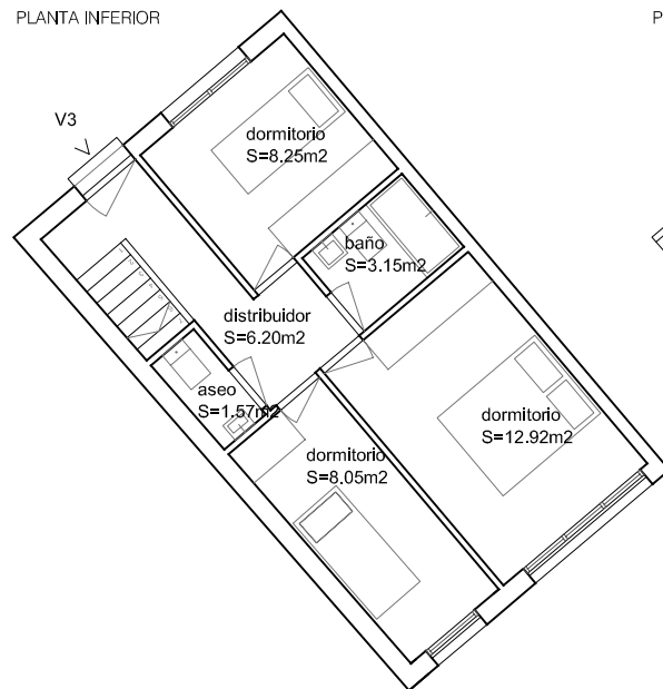
PLANTA INFERIOR
