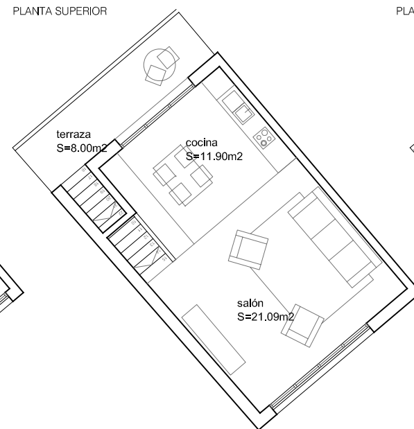
PLANTA SUPERIOR
