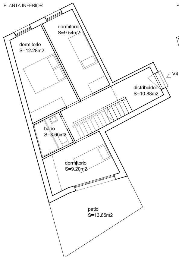
PLANTA INFERIOR
