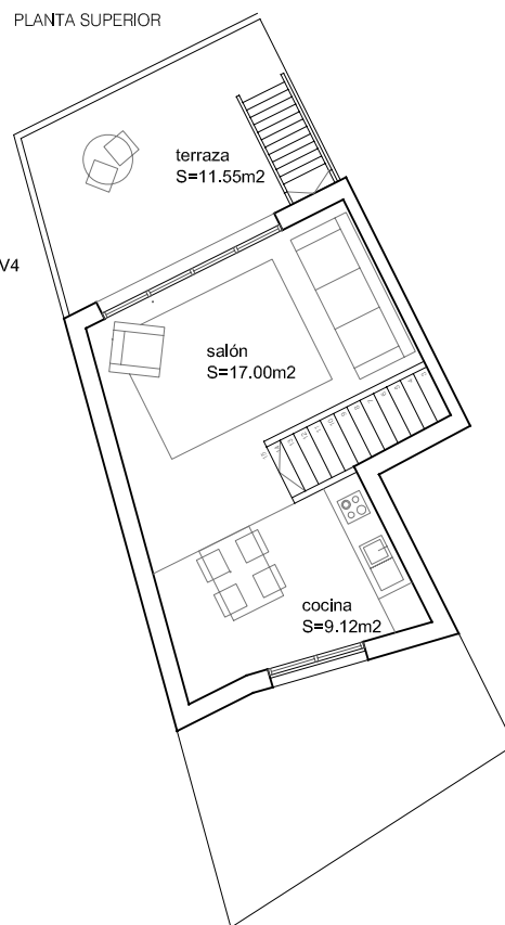
PLANTA SUPERIOR
