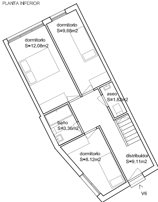
PLANTA INFERIOR
