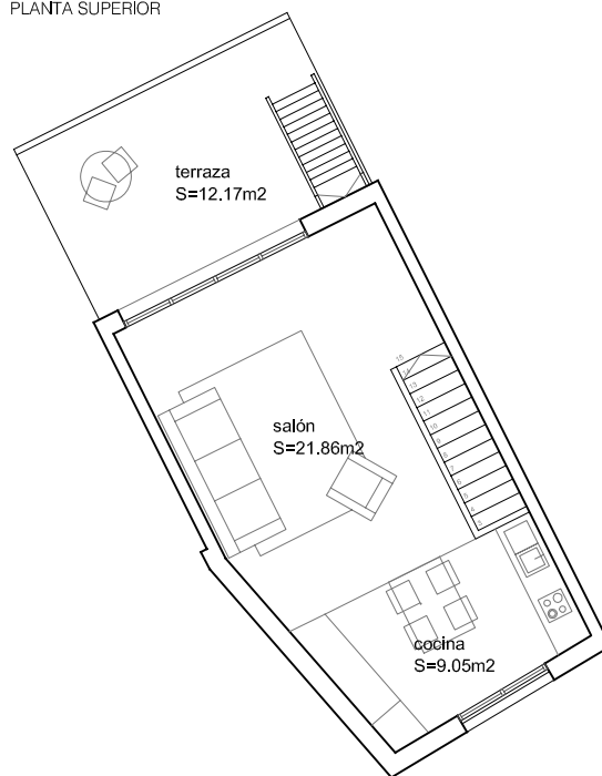
PLANTA SUPERIOR
