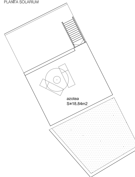
PLANTA SOLARIUM
