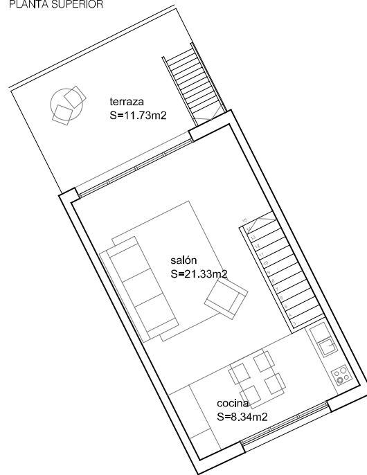
PLANTA SUPERIOR
