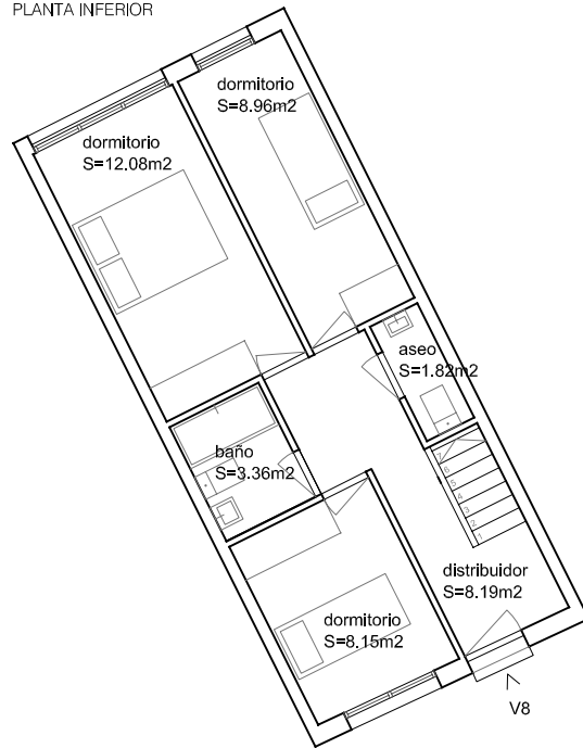
PLANTA INFERIOR
