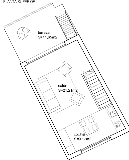
PLANTA SUPERIOR
