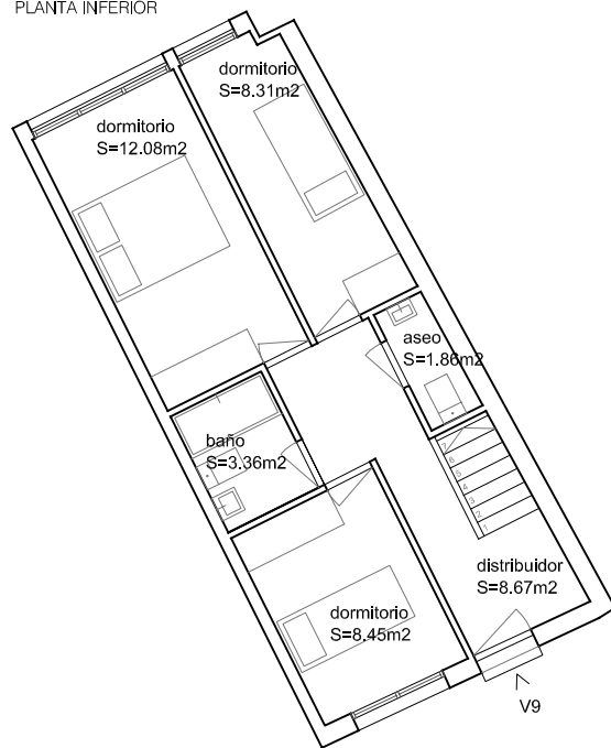
PLANTA INFERIOR
